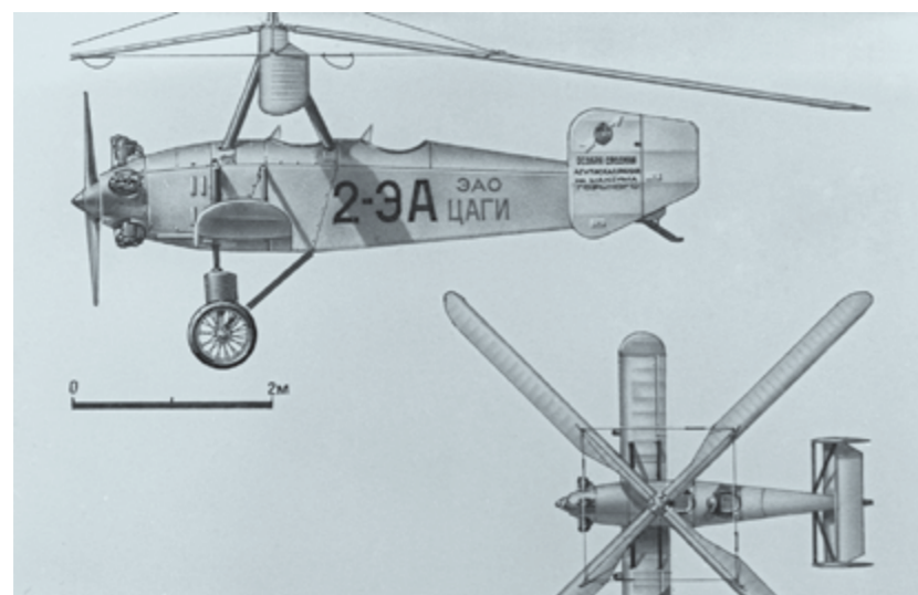
АВТОЖИР ЦАГИ 2-3А – ДВУХМЕСТНЫЙ АППАРАТ С ДВИГАТЕЛЕМ «ТИТАН» МОЩНОСТЬЮ 230 л.с. ПЕРВЫЙ ПОЛЕТ ОСУЩЕСТВЛЕН В 1931 ГОДУ
