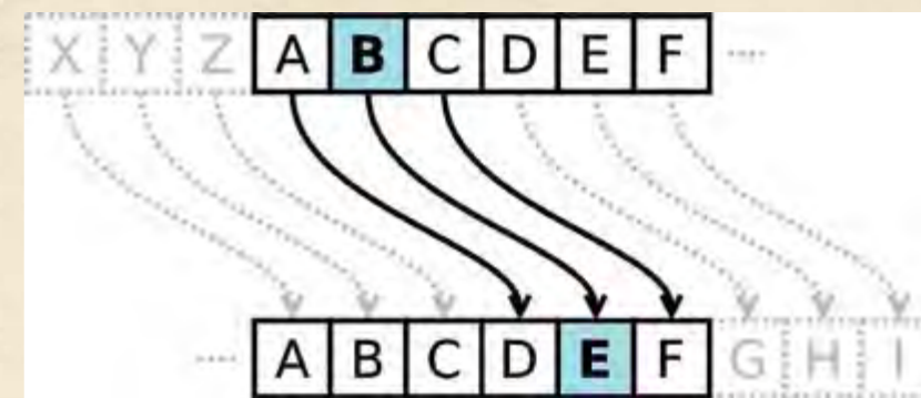
ШИФР ЦЕЗАРЯ: ПРИ ШИФРОВАНИИ КАЖДЫЙ СИМВОЛ ЗАМЕНЯЕТСЯ ДРУГИМ, ОТСТОЯЩИМ ОТ НЕГО В АЛФАВИТЕ НА ФИКСИРОВАННОЕ ЧИСЛО ПОЗИЦИЙ
