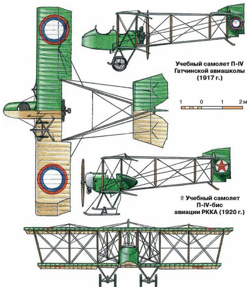
САМОЛЕТ П-IV ПРЕДНАЗНАЧАЛСЯ ДЛЯ ПЕРВОНАЧАЛЬНОГО ОБУЧЕНИЯ ЛЕТЧИКОВ
