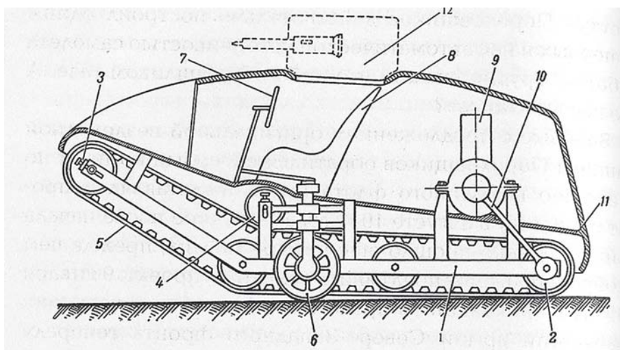
СХЕМАТИЧЕСКИЙ РАЗРЕЗ «ВЕЗДЕХОДА» [ЖУРНАЛ ТАНКИСТ 1952 Г.]
